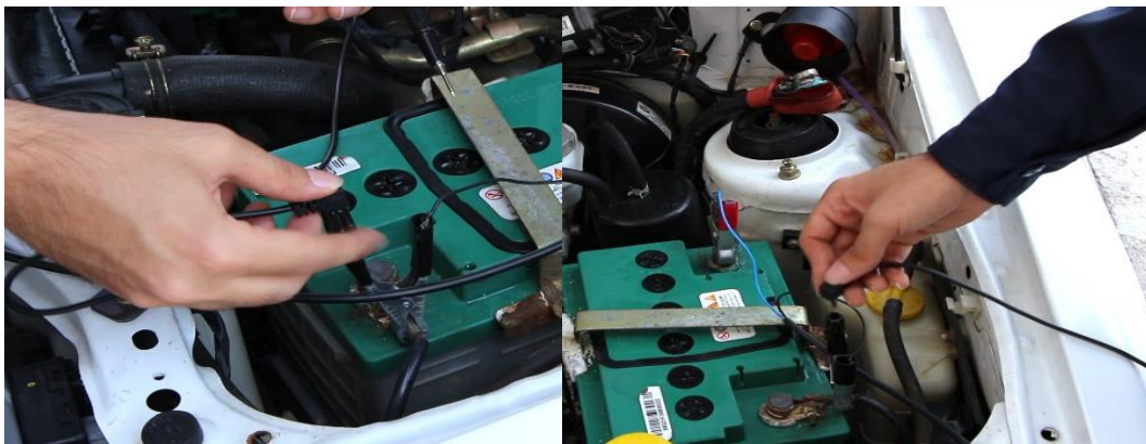
نصب پروب رابط به گیره سوسماری
